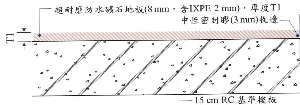
(b)A-A'剖面示意圖
