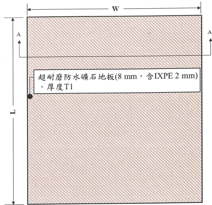
(a)試件平面示意圖
