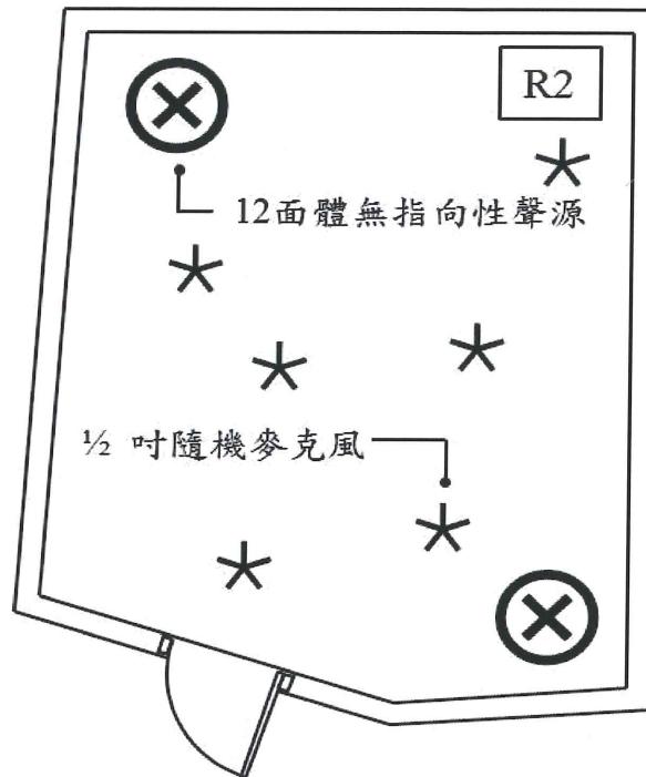
圖4.1 試驗設備配置平面示意圖
